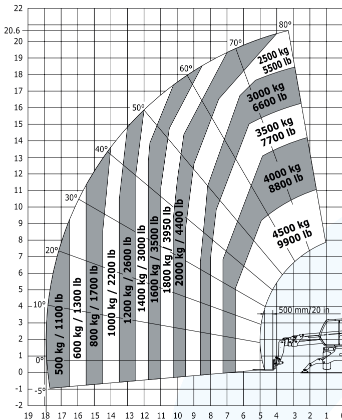
diagrama de capacidade [sobre estabilizadores]
